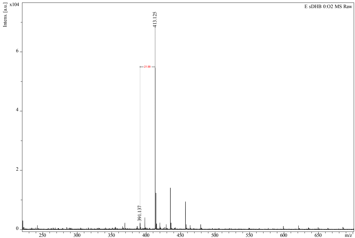
MALDI-TOF спектр; рефлексный режим положительных ионов, матрица ДНВ; молекулярный ион имеет массу 391.15 m/z [M+H + ], однако на спектре преобладает ион с массой 413,12 m/z [M+Na + ].
